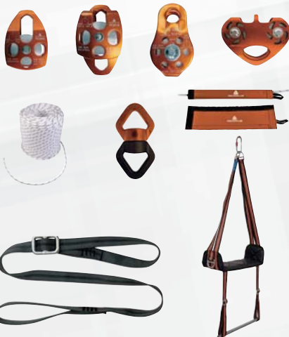
EN 1891 CORDE
